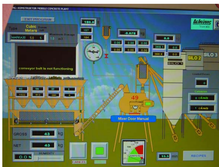
Izgled monitorskog prikaza rada vage
